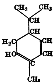
\alpha -Phellandrene.
